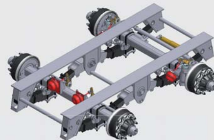
Pevný nebo natáčecí snížený tandem
