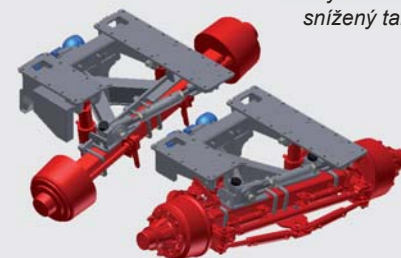
Pevné nebo natáčecí odpružení typu Delta
